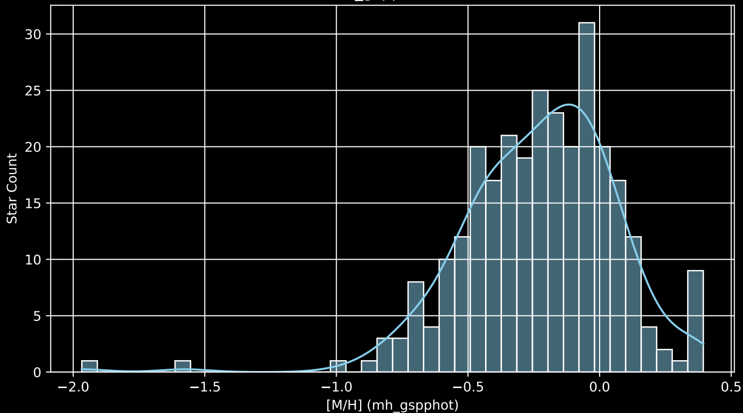
GALAH DR4 Field: [647] [M/H] (mh_gspphot) (n= 285)
