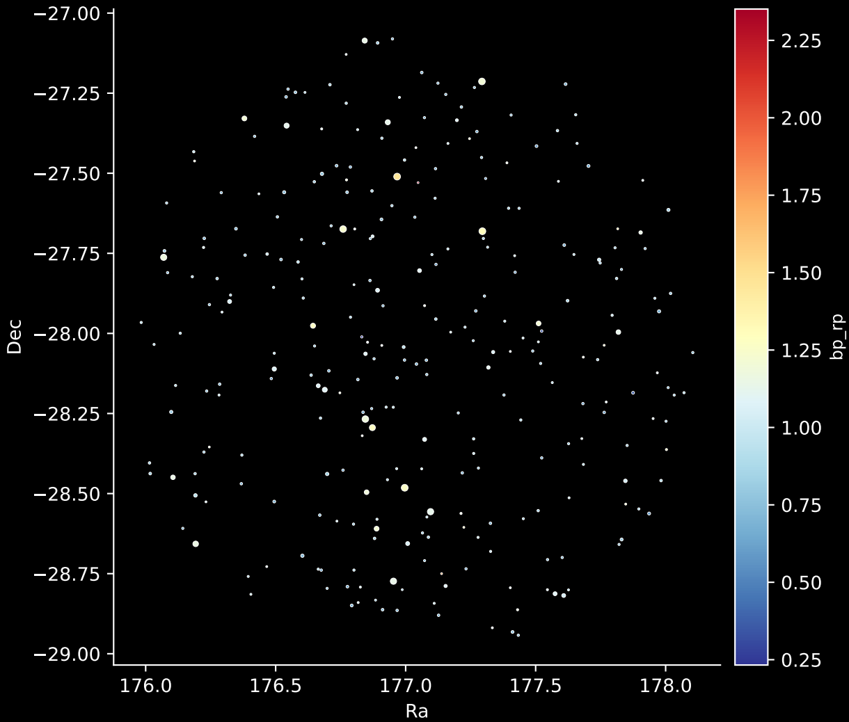
GALAH DR4 Field: [647] Stars: 287
