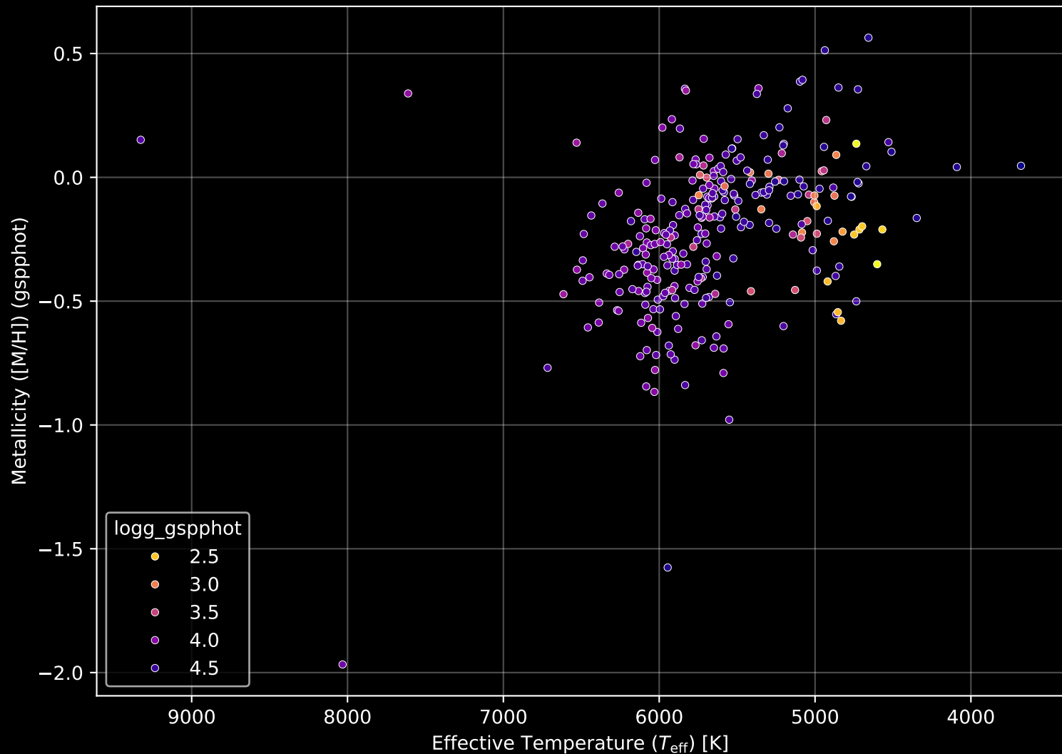
GALAH DR4 Field: [647] Stellar Population Parameters (n= 287)
