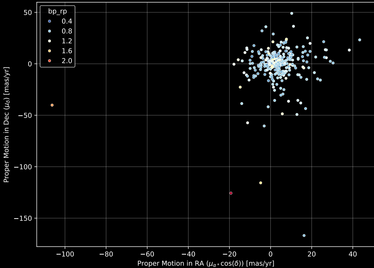
GALAH DR4 Field: [647] Proper Motion Diagram (n= 287)
