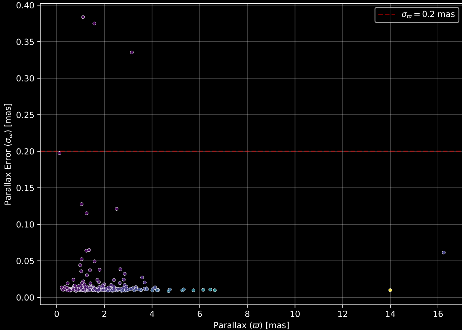
GALAH DR4 Field: [647] Parallax Quality (n= 287)
